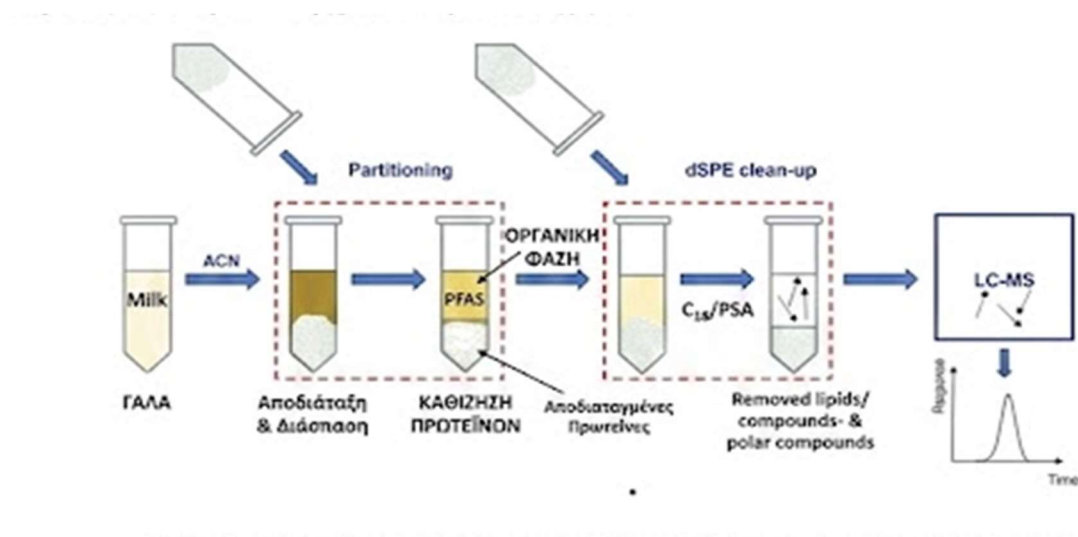
Σχήμα 14: Αναπαράσταση της μεθόδου QuEChERS ( Godfrey, et al., 2020)
