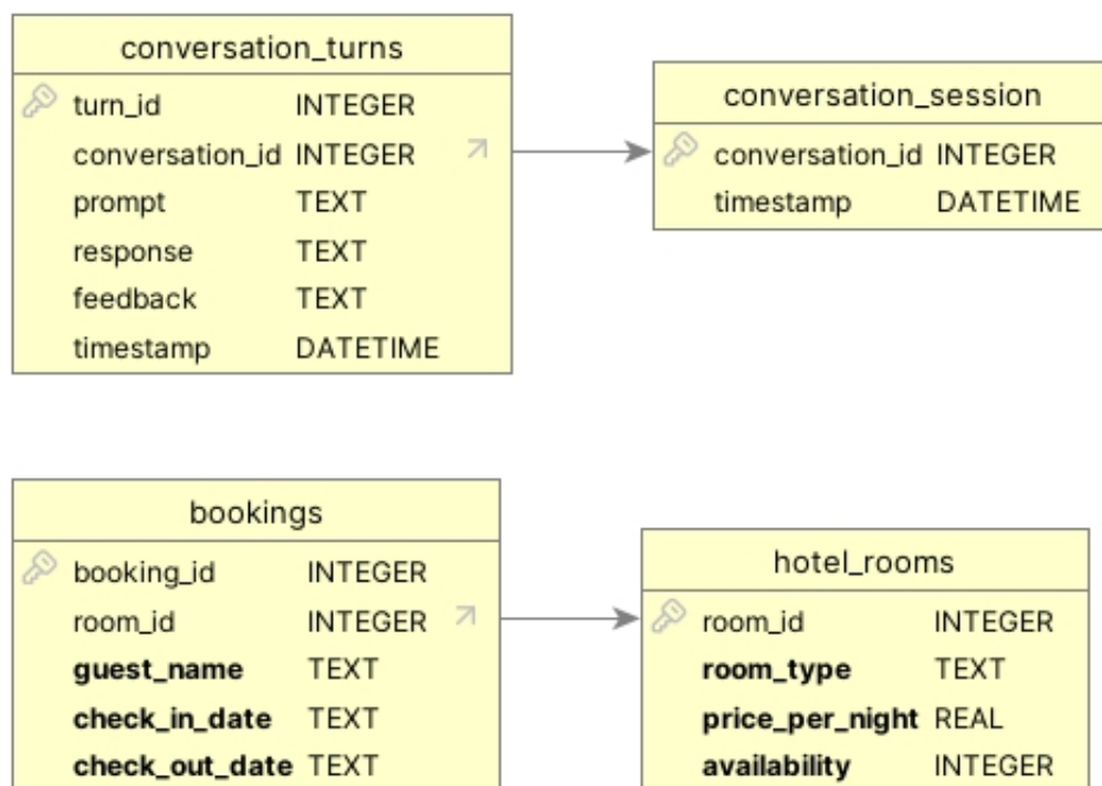
Εικόνα 17 : Διάγραμμα οντοτήτων-συσχετίσεων
